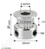
20T W6 B6.35 Poulie GT2 - courroie 6mm dents 20 axe 6.35mm 15 DH
