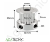
20T W7 B4 Poulie GT2 - courroie 7mm dents 20 axe 4mm 16 DH
