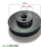
Poulie GT2 6mm 60 dents 8mm 45 DH
