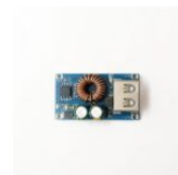
QC-MINI MODULE DE CHARGEUR CC USB
