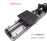
kit linéaire axe Z 300mm, nema 23 pour machine cnc 3500 DH
