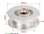
Poulie GT2 20 sans dents qualite D=5mm*10mm 16 DH
