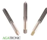
tarauts à filetage manuel M6 x 1,0 mm 50 DH
