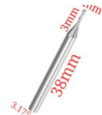
3mmxD1x3x38mm Fraise en carbure à simple cannelure pour aluminium CNC 80 DH
