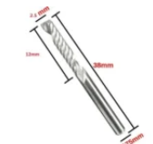
3.17xD2.5x12x38mm Fraise en carbure à simple cannelure pour CNC 13.5 DH
