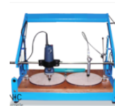
duplicateur de sculpture sur bois, machine à copier des formes en bois 9500 DH
