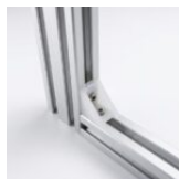
Equerre en plastique pour Profilés Aluminium T-Slot V-slot-20*20-M4
