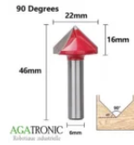
Mèches V de router à tige de 6*22*90 degré 60 DH
