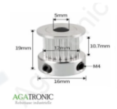
20T W10 B5 Poulie GT2 - courroie 10mm dents 20 axe 5mm 16 DH
